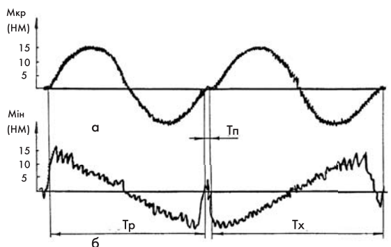
Рис. 3. Копії осцилограм крутних моментів
