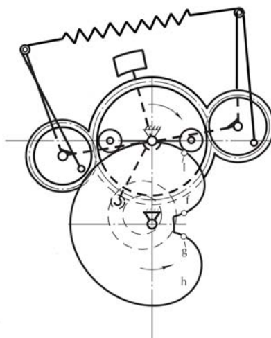
Рис. 1. Кінематична схема напівкривошипного механізму
