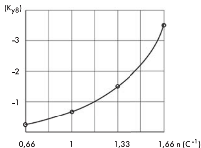
Рис. 8. Графік залежності коефіцієнтів зрівноваження
