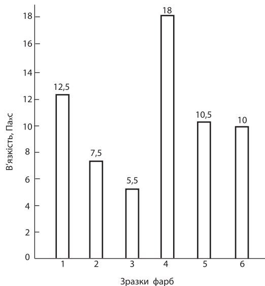
Рис. 1. В'язкість модельних зразків фарби: 1 — мф1; 2 — мф2; 3 — мф3; 4 — мф4; 5 — мф5; 6 — мф6
