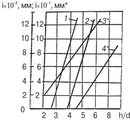
Рис. 2. Вплив відносної довжини приєднуваної деталі h/d на величину складального зазору i для d = 2^\circ ; S = 1,5 ; f = 0,15 .
