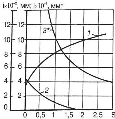
Рис. 4. Вплив відносного зусилля складання S на величину складального зазору ( \alpha = 2^\circ , f = 0,15 і h/d = 4 ). 1 — установка вала під втулку, \beta = 0^\circ ; 2 — установка втулки на вал, \beta = 0^\circ ; 3 — установка втулки на вал, \beta = 90^\circ
