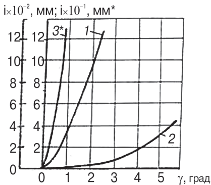
Рис. 3. Вплив точної характеристики складального верстата a на величину складального зазору f = 0,15 ; h/d = 4 , S = 1,5 . 1 — установка вала під втулку, \beta = 0^\circ ; 2 — установка втулки на вал, \beta = 0^\circ ; 3 — установка втулки на вал, \beta = 90^\circ
