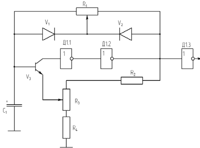
Рис. 3. Схема ГНЧ
