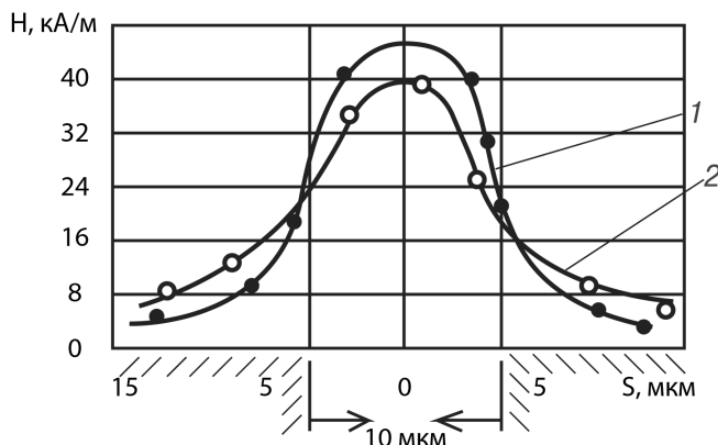
Рис. 7. Горизонтальна складова напруженості H магнітного поля ( S = 10 мкм) при надтонкій абразивній обробці композитних матеріалів на основі інструментальної сталі 5ХЗВЗМФС: 1 — прецизійна машинна доводка на чавунних притирах послідовно мікропрошарками електрокорунда хромчастого зі змістом у складі оксиду хрому CrO до 2 % послідовно 33АМ5, 33АМ3 і 33АМ1; 2 — тонке абразивне шліфування кругом з карбїду кремнія зеленого на гліфталевій зв'язці — 63СМ14СМ2ГЛ
